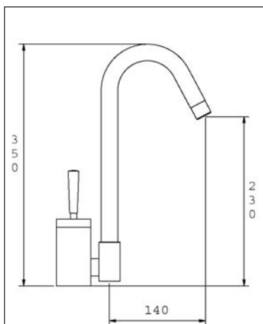
BM FX73CH
