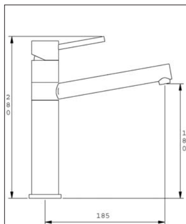
BM FX200CH
