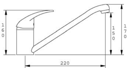
BM FX71CH
