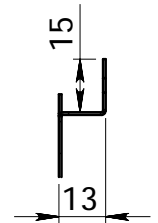
C 比例 1:2
