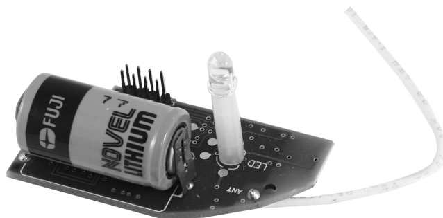
Ei605MTYRF Module
